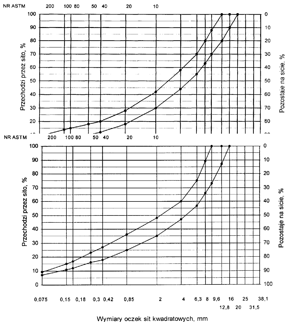
Rys. 1. Krzywe graniczne uziarnienia mieszanki mineralnej BA od 0 do 12,8 mm do warstwy ścieralnej nawierzchni drogi o obciążeniu ruchem od KR2 do KR6
